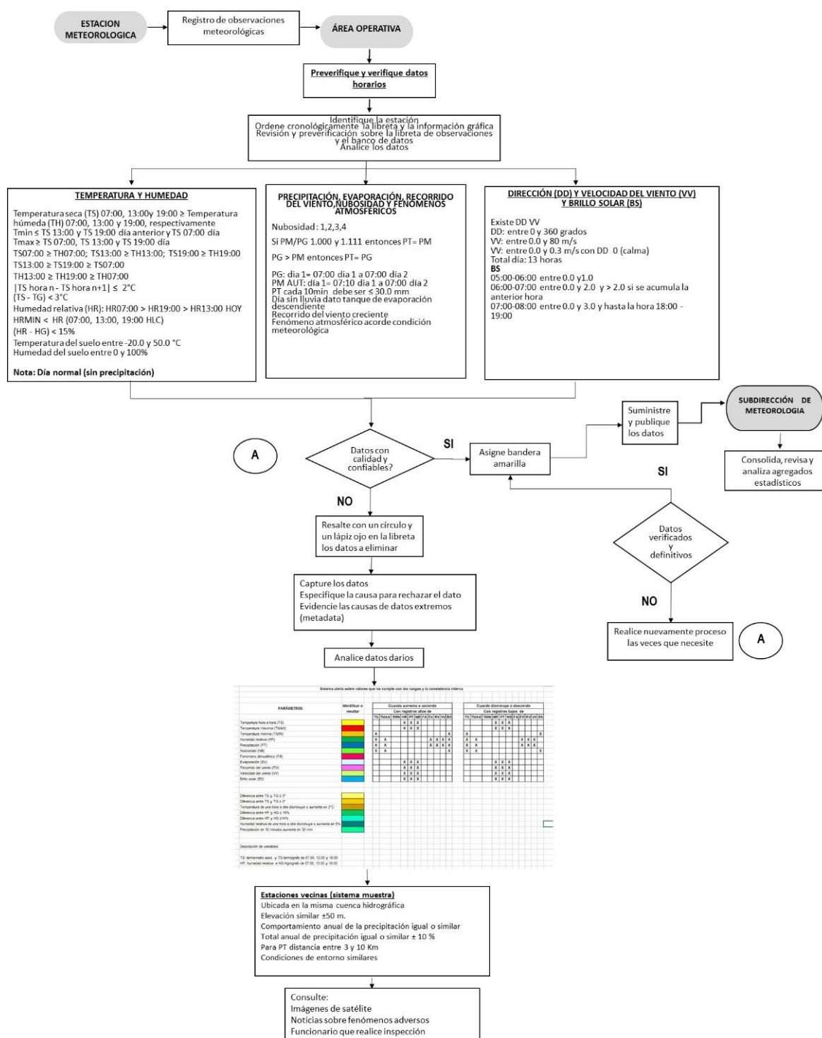
Figura 1. Diagrama de flujo de la información para la gestión de datos Meteorológicos
