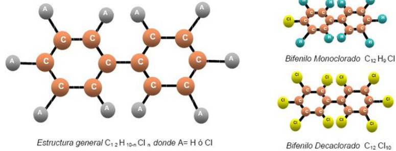
Figura 1. Estructura molecular de los PCB
